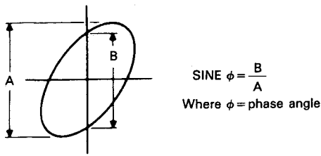
Fig. 46 Phase shift calculation
